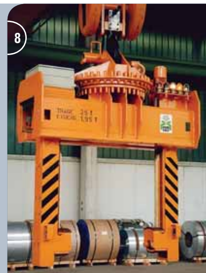
8 Elektromotorischer Teleskopcoilgreifer mit Horizontaldrehwerk, mit Lichtschranken zur Erfassung des Coillinnendurchmesser. Electromotive telescopic coil grab with horizontal slewing gear, with light barriers to detect the coils eye.
