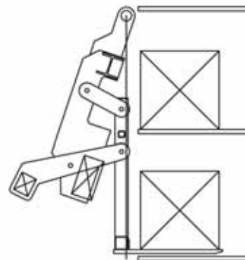
4 Aufnahmestellung Lifting position
