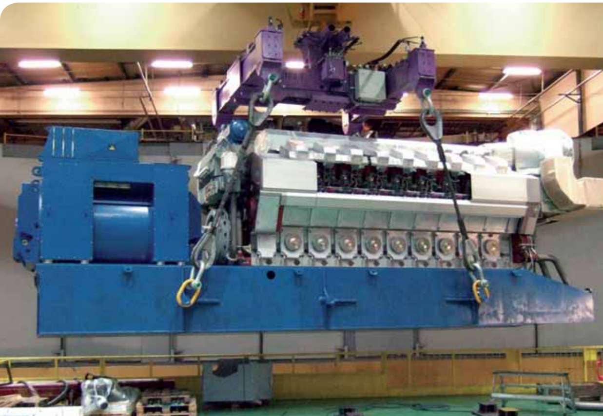
Schwerlasttraversen Wendevorrichtungen
